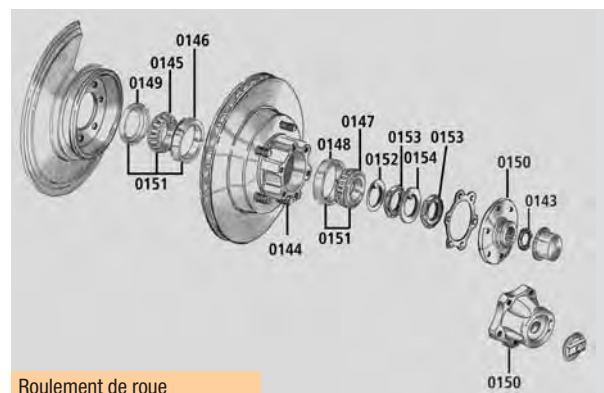
Roulement de roue
