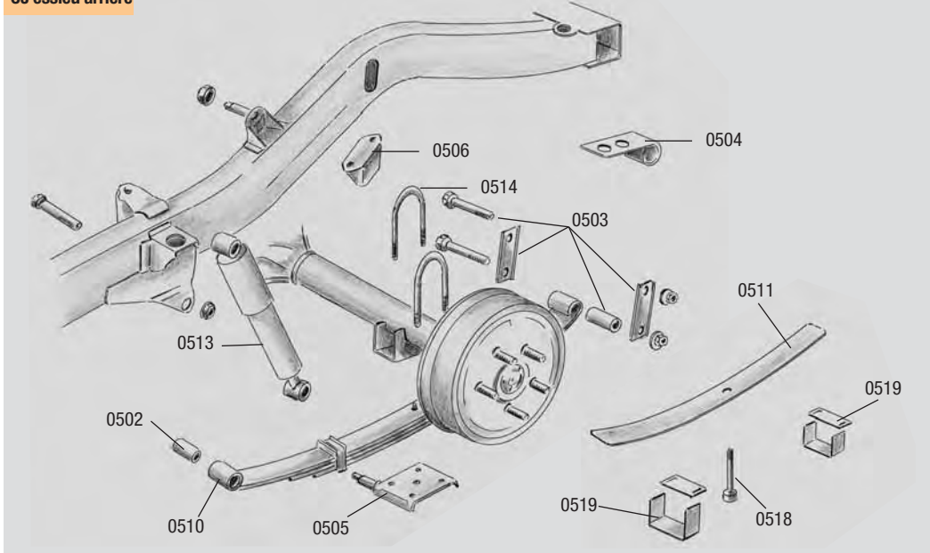
CJ essieu arrière
