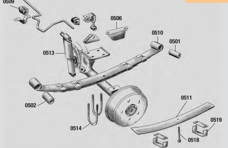
Essieu arrière XJ
