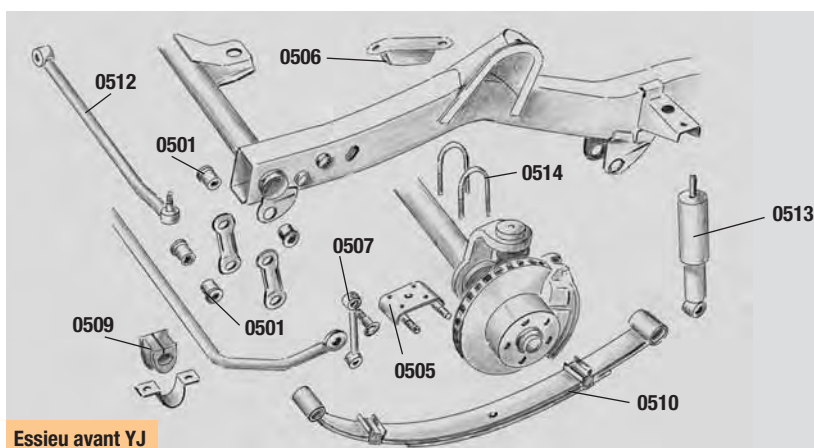
Essieu avant YJ
