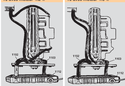
YJ avec moteur 4.2-l.
